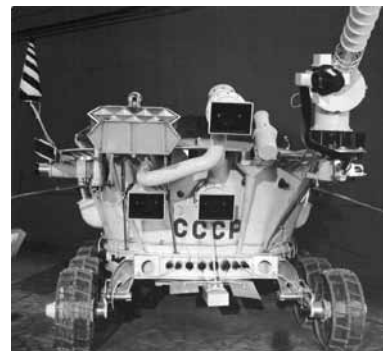
Луноход-2
